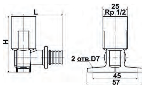
Водорозетка аксиальная удлиненная
