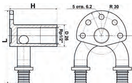
Водорозетка аксиальная проходная
